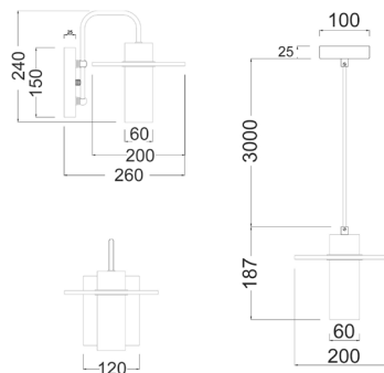
LUCERNA-W1 (Wall Light)
